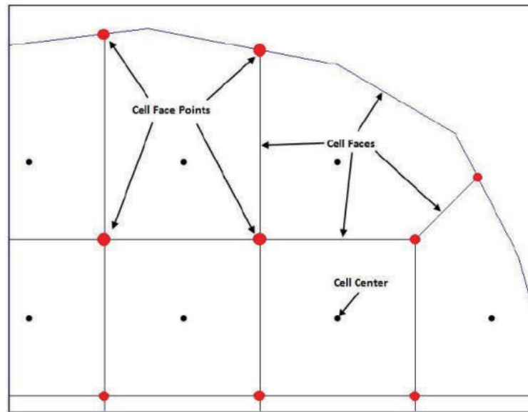
Fig. 5.1 - Esempio mesh computazionale HEC-RAS 5.0.6
